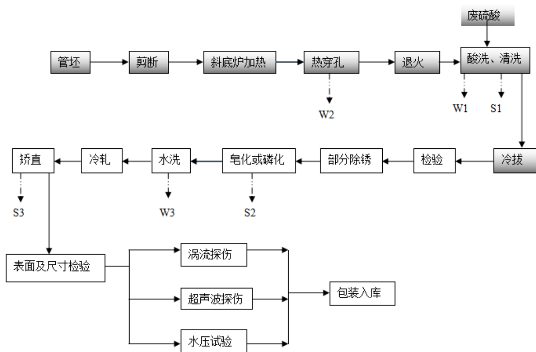
图 2.2-1 生产工艺流程图
