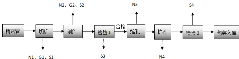
图 2.2-2 生产工艺流程图
