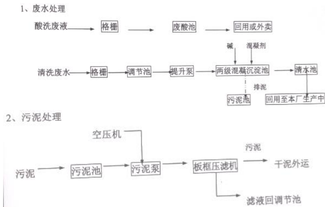
图 2.2-5 废水预处理工艺流程图
